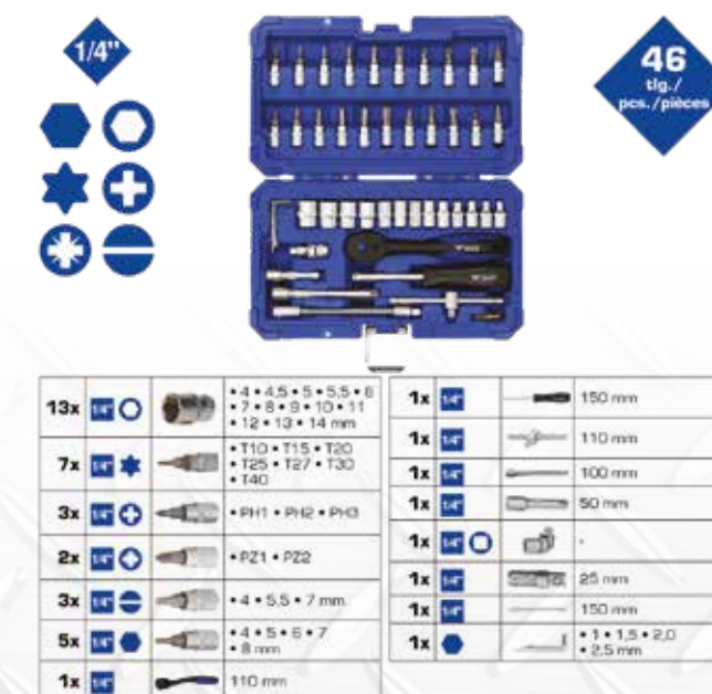
1/4" SET UTIČNIH KLJUČEVA, 46-DIJELNI šifra BT020046
